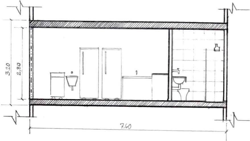
CORTE AB 1:75
