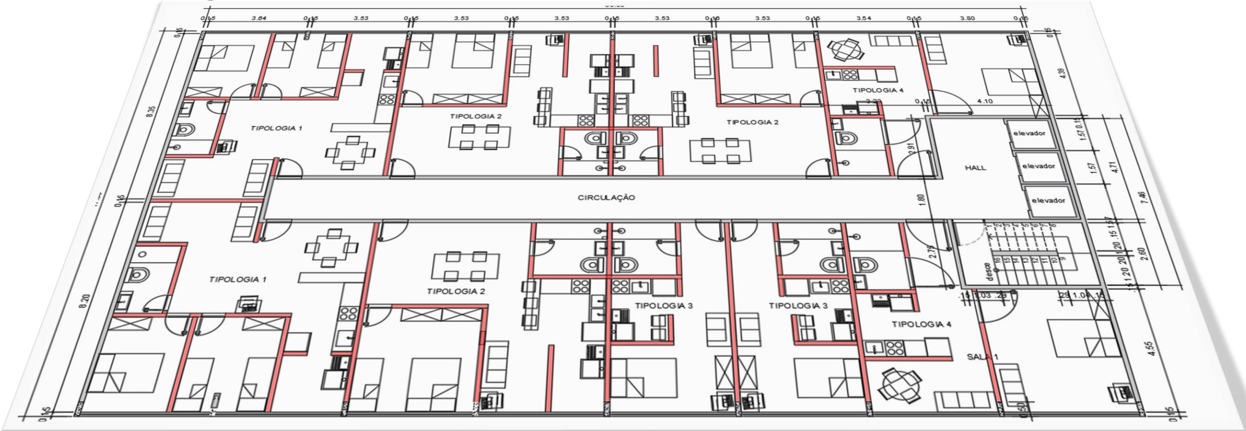
PLANTA PAVIMENTO TIPO ESC. 1/125
